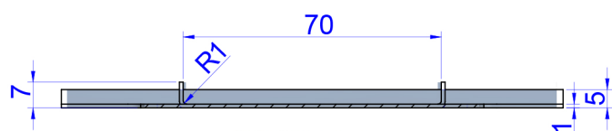
CORTE A-A
